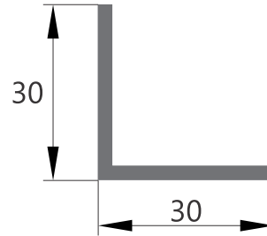
L30x30 Elox, Bela
